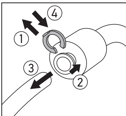
Последовательность действий при отсоединении шланга (патрубка): 1 - извлечь; 2 - утопить ключом; 3 - вытянуть рукой; 4 - вставить.
