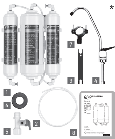
Рис.3. Комплект поставки фильтра Econic Osmos Stream.
