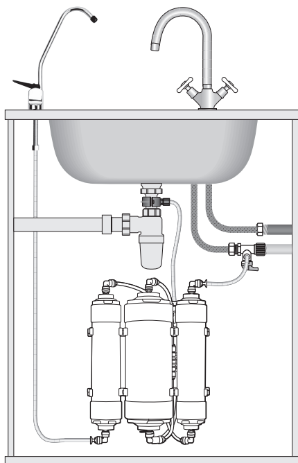
Рис.1. Пример установки фильтра Econic Osmos Stream.
